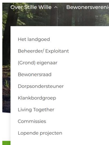
Afbeelding 2: menustructuur
